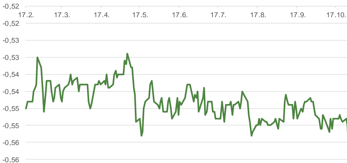
Euribor 3M
