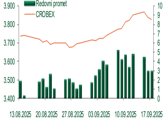
Kretanje vrijednosti CROBEX-a i redovnog prometa
